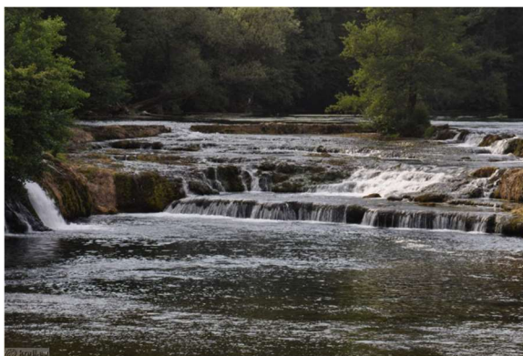
Slika 14: Lehnjakovi pragovi v Žužemberku
